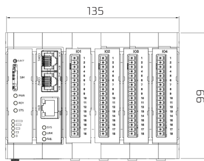
Wymiary mechaniczne wersji rozszerzonej
