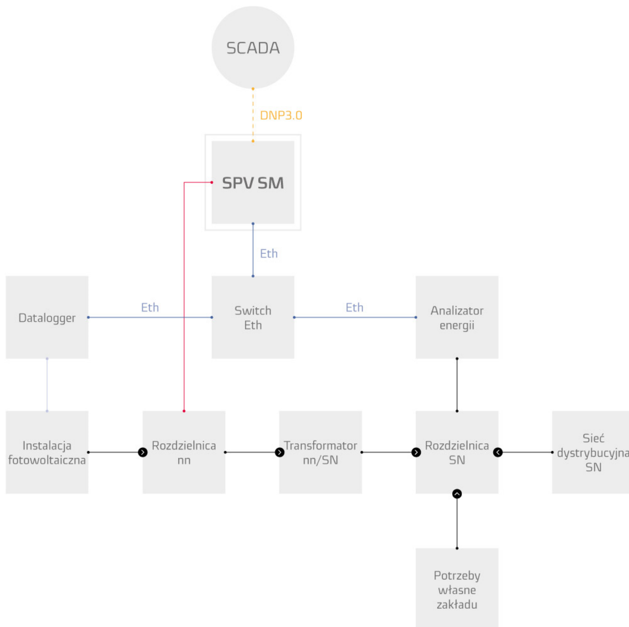
Rys. 1. Przykład zastosowania sterownika SPV SM
