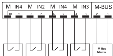
Wersja 1: M-BUS + 4 wejścia imp.
