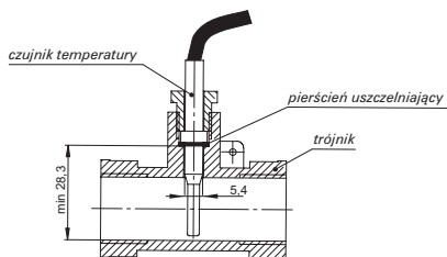
Montaż czujnika w trójniku
