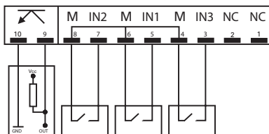
Wersja 4: 3 wejścia imp. + 1 wyjście imp.
