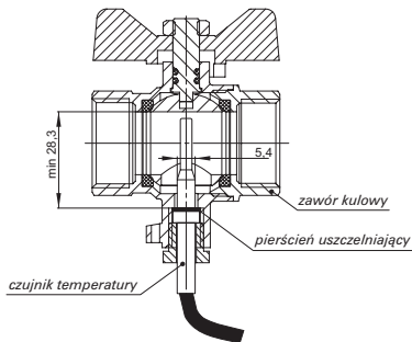
Montaż czujnika w zaworze kulowym
