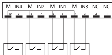
Wersja 3: 4 wejścia imp.
