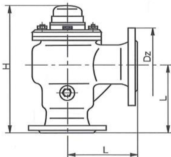
Ilustracja nr 3. Wymiary instalacyjne
